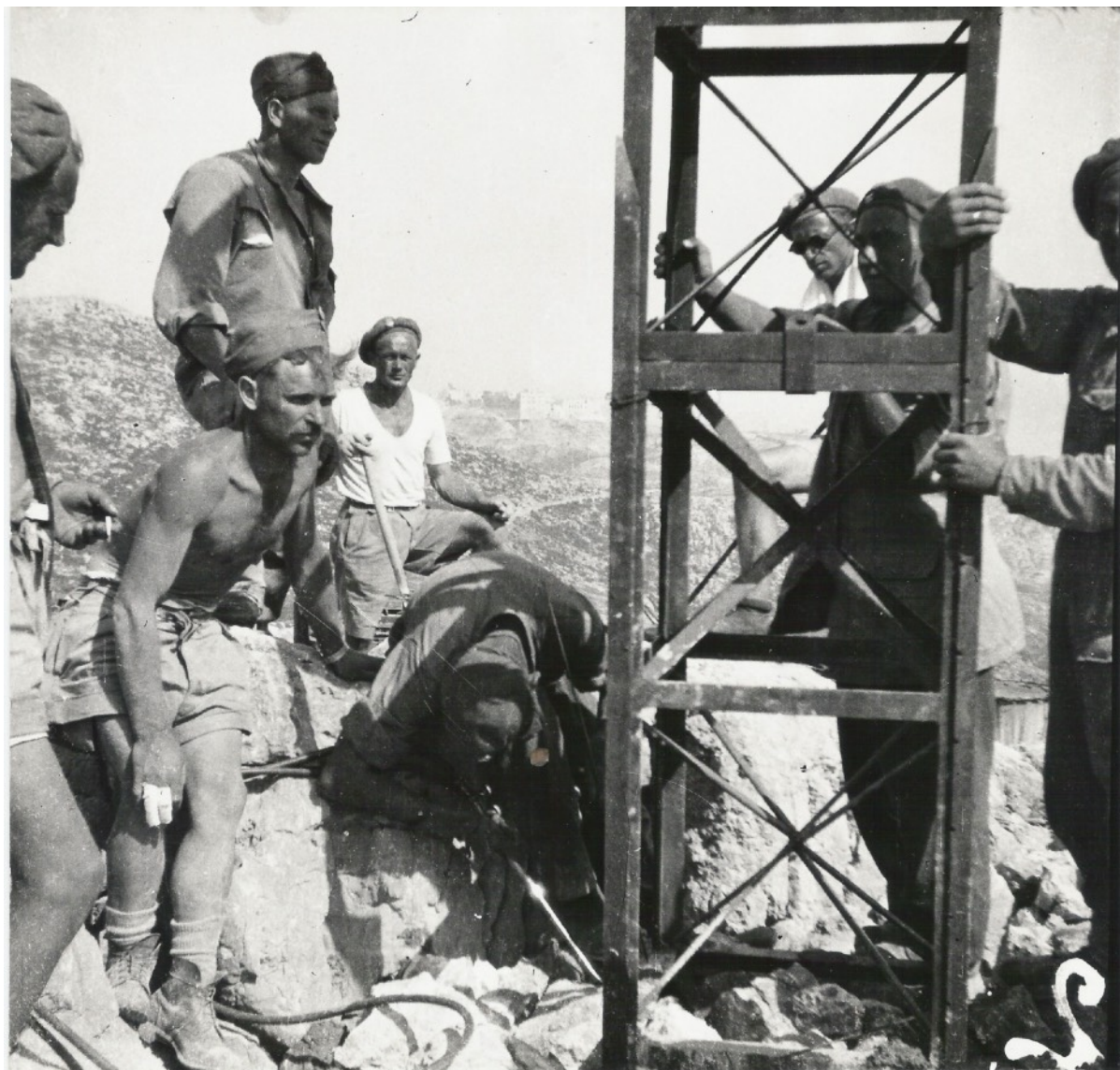
Fot.2. Dodatkowe wzmocnienie konstrukcji podstawy (dospawanie w narożach kątownika), pionowanie i zafundamentowanie. W głębi zdjęcia widoczny klasztor M. Cassino. Za kratownicą stoją: por. Waław Kulikowski – dowódca grupy (w okularach) i plut. Bolesław Abramczyk. Maj 1944 r. (III dekada).
